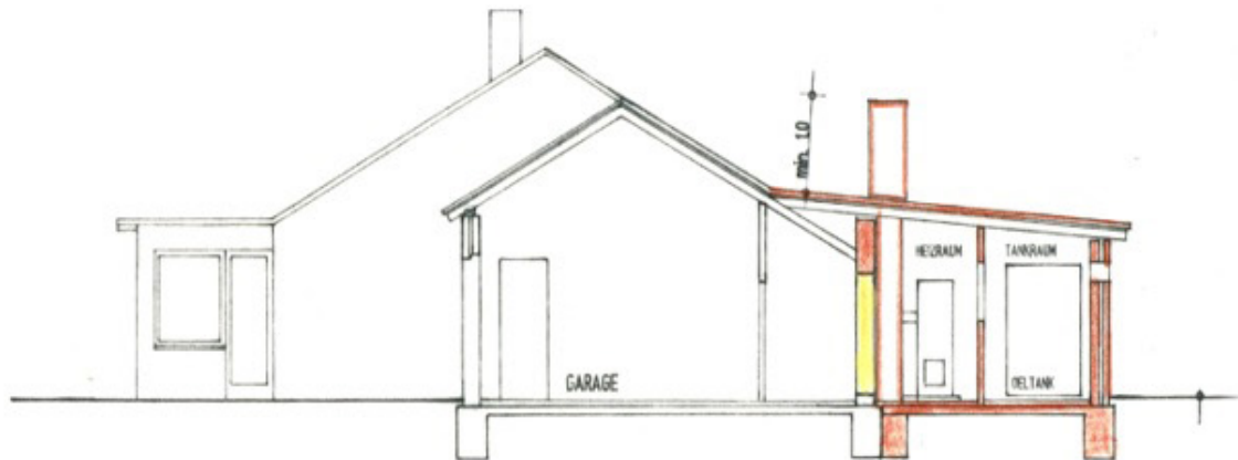
SCHNITT A-A
