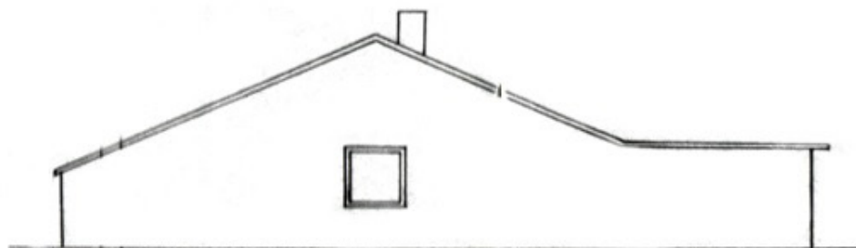
Nordwest-Ansicht
